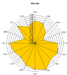
Grafico 3.4 - Coefficienti di correlazione per i delitti legati alle organizzazioni malavitosi
